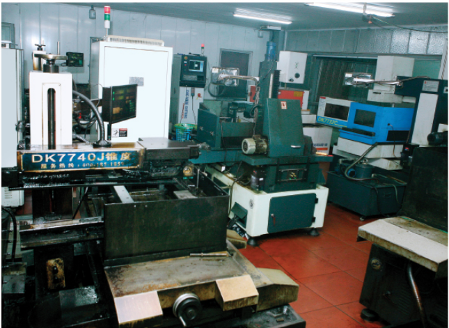
Máy cắt dây/ ワイヤー切断機
